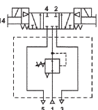
Общий регулятор отверстий с 4-ходовым, 3-позиционным клапаном АРВ соленоидным клапаном АРВ
