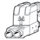
Типоразмер 2 4/3 все отверстия блокированы P2M2SBEE2CV2AF0
