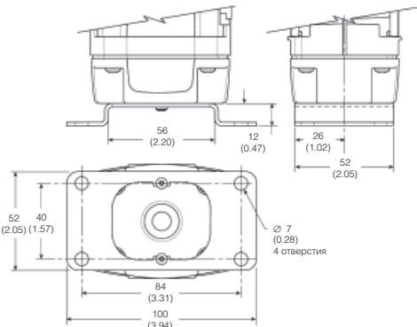
Напольный кронштейн
