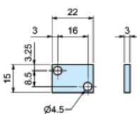
Прижимная планка, P2LA
