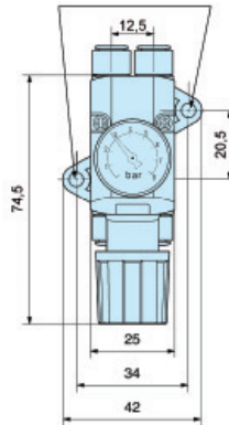
Крепление 2 винтами диаметром 4 мм на убираемых кронштейнах
