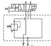
Избирательный регулятор с 4-ходовым, 2-позиционным одиночным соленоидным клапаном
