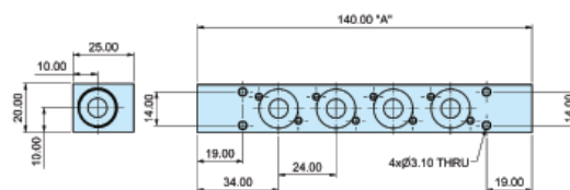
Прижимная планка, P2LB
