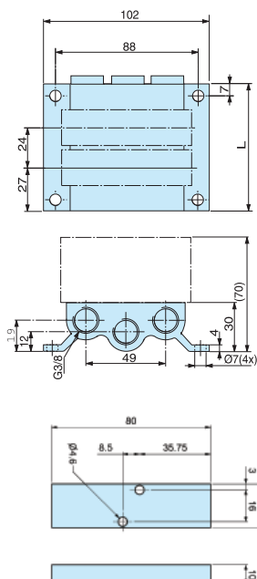
Прижимная планка, P2LA
